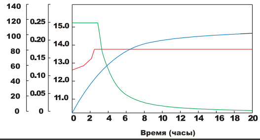
Заряд постоянным напряжением (0.3СА, 25°C)
