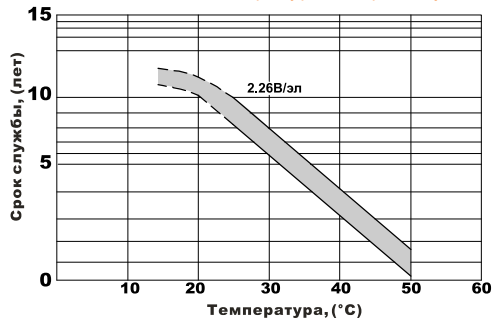
Влияние температуры на срок службы
